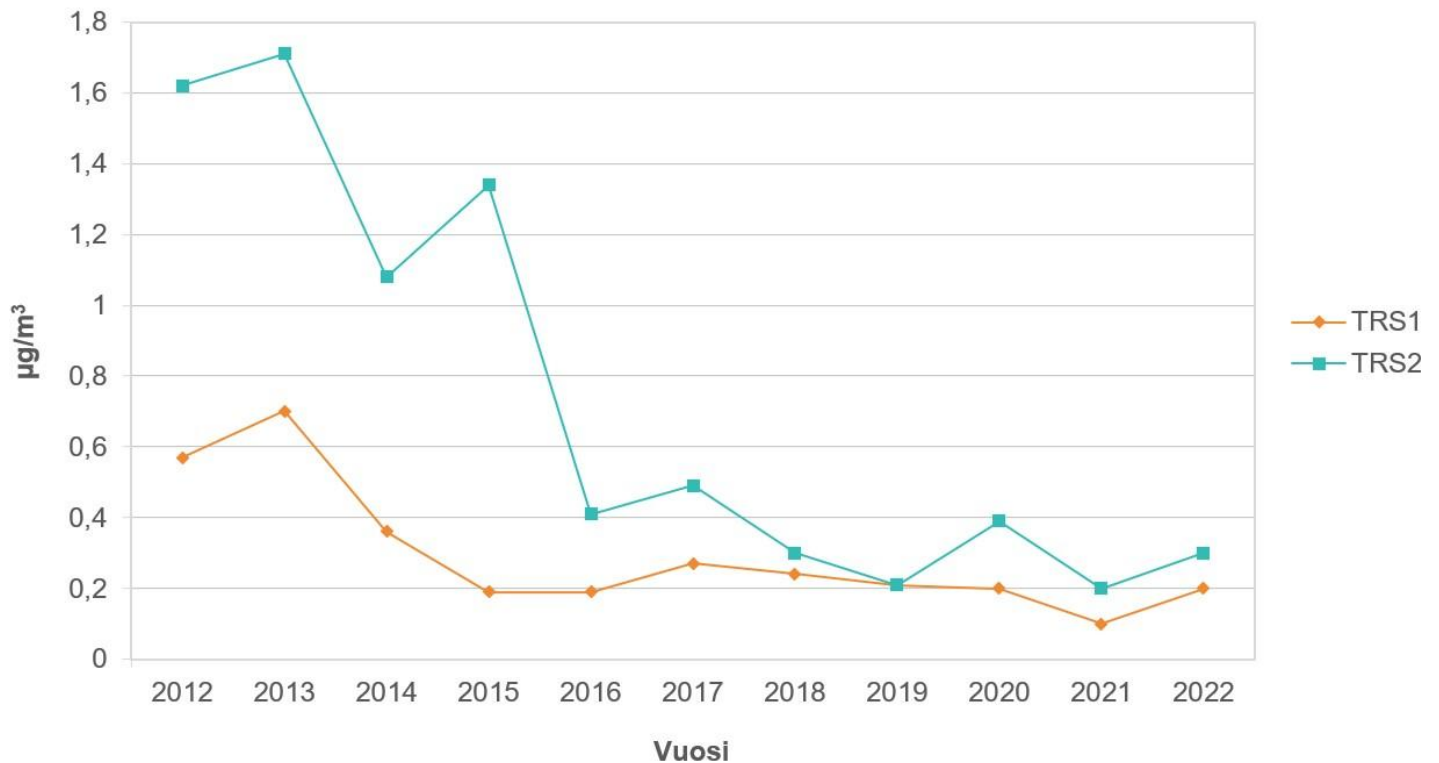
Kuva 13. Haisevien rikkiyhdisteiden (TRS) pitoisuuksien (µg/m³) vuosikeskiarvot ilmanlaadun mittausasemilla 1 (TRS 1) ja 2 (TRS 2) vuosina 2012–2022.
