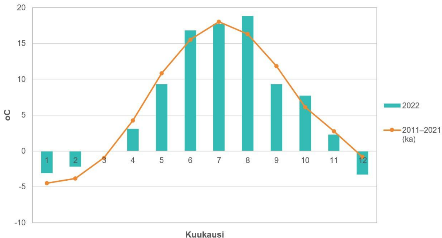
Kuva 10. Kuukausittaiset keskilämpötilat (°C) Ämässuon jätteenkäsittelykeskuksen sääasemalla sekä vuonna 2022 että vuosina 2011–2021 (keskiarvo, ka).
