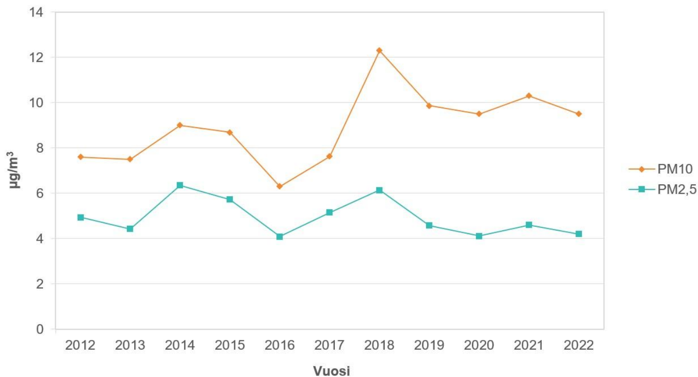
Kuva 12. Ämmässuolla mitattujen hengitettävien hiukkasten (PM10) ja Ämmässuolla mitattujen pienhiukkasten (PM2,5) vuosikeskiarvot ( \mu\text{g}/\text{m}^3 ) vuosina 2012–2022.
